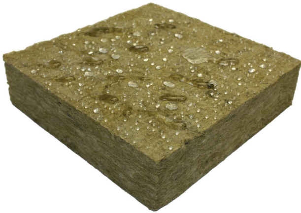
Figure 4. Isolant continu en laine minérale RainBarrier MD avec résistance à la compression élevée
